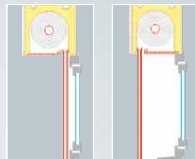
Tunnelmontage buitenoprolling
